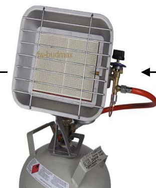
Ogrzewacz gazowy
